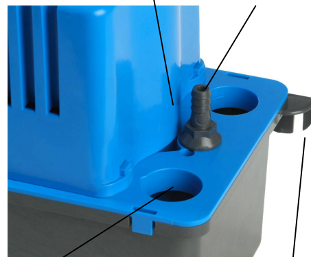
Integriertes Rückschlagventil
